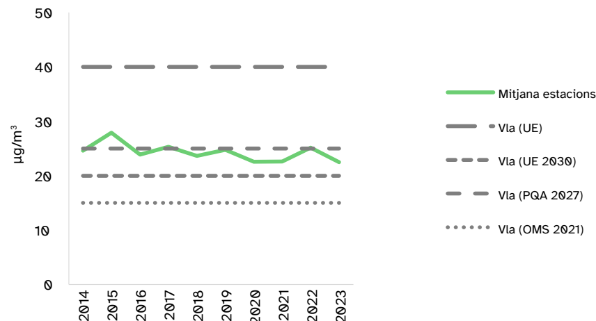
Nivells d'immissió de PM 10 (mitjana anual) i valors límits anuals (Vla) per diferents normatives. AMB, 2014-2023.
