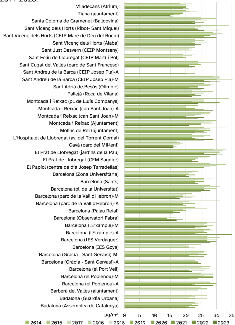
Concentració mitjana anual de PM 10 per estacions. AMB, 2014-2023.
