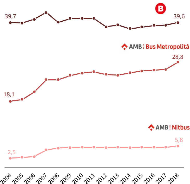
Oferta en veh-km (milions); 2004-2018
