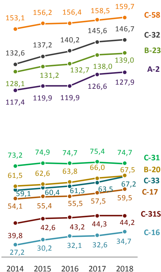
Intensitat mitjana diària (dll. – dj.) a les vies d'alta capacitat de l'àrea metropolitana de Barcelona (milers). 2014 - 2018
